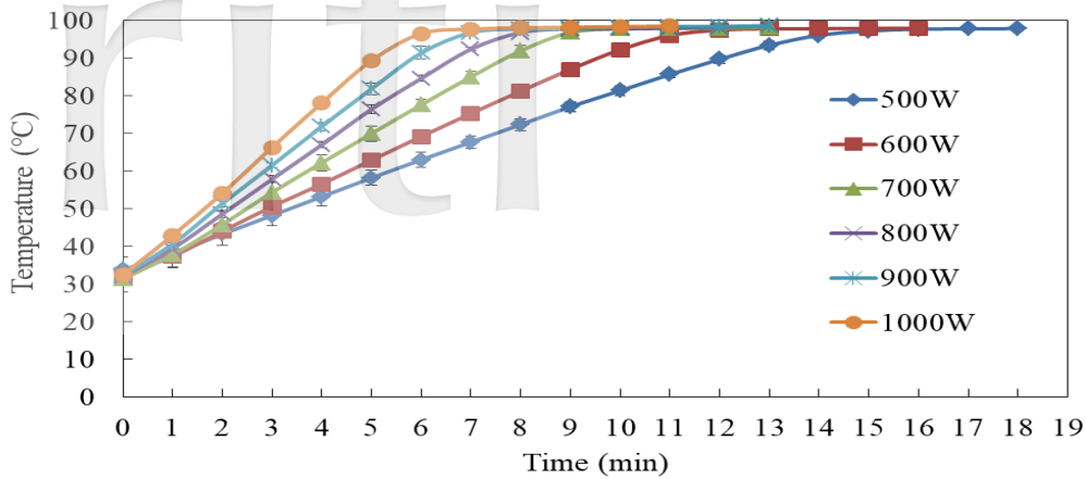
圖 1. 不同微波功率之 500 mL 水的升溫曲線。
